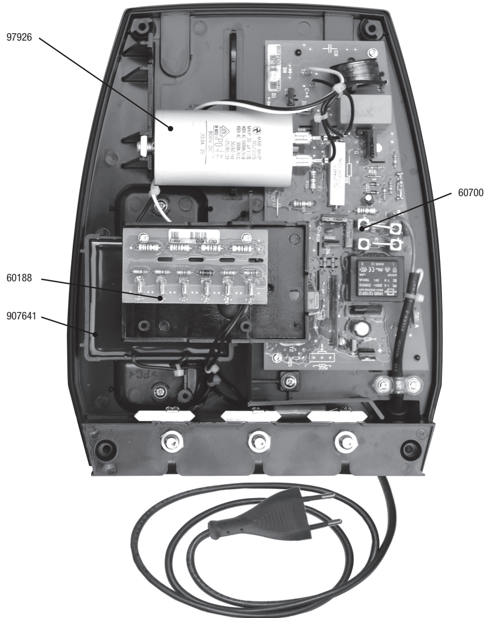
Fig. 1 Ersatzteile | Spare parts | Pièces détachées | Peças Pezzi di ricambio Reservedele | Reserve onderdelen | Alkatrészek | Części zapasowe
